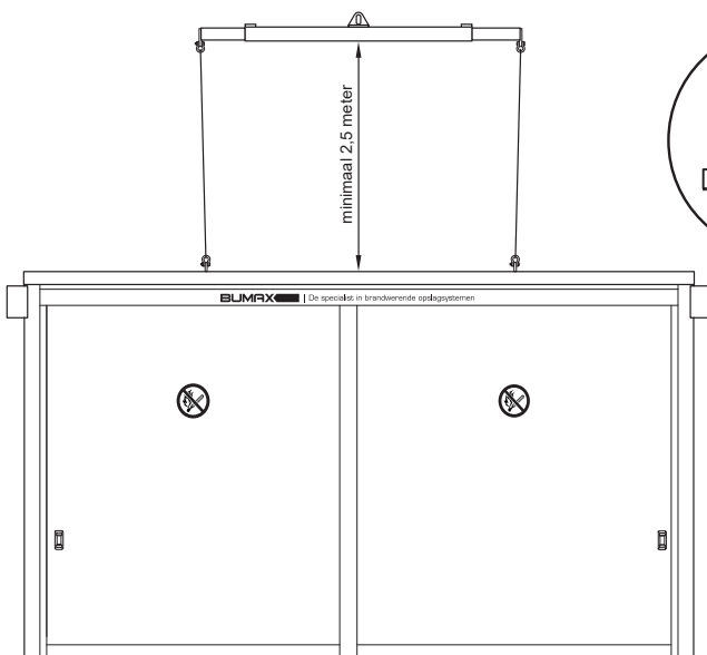
Hijshoogte minimaal 2,5 meter
