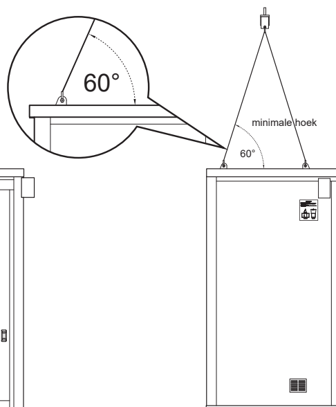
Hoek van de hijsbanden minimaal 60°
